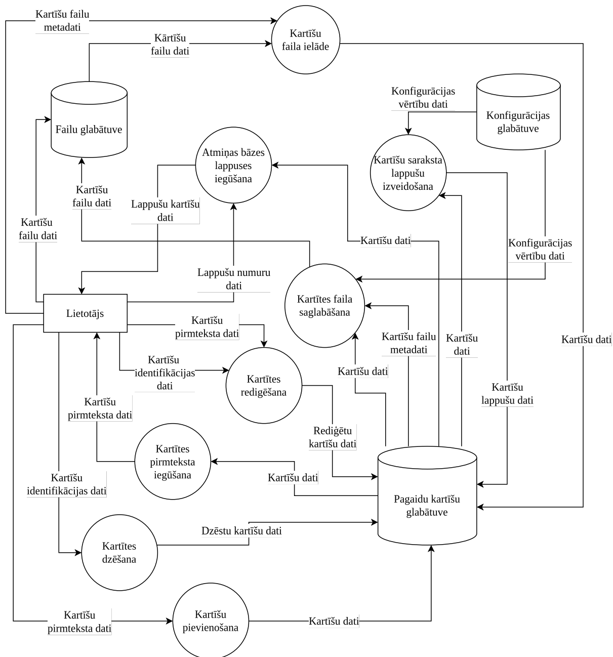
2.2. att. Atmiņas bāzes moduļa 2.līmeņa datu plūsmas diagramma
